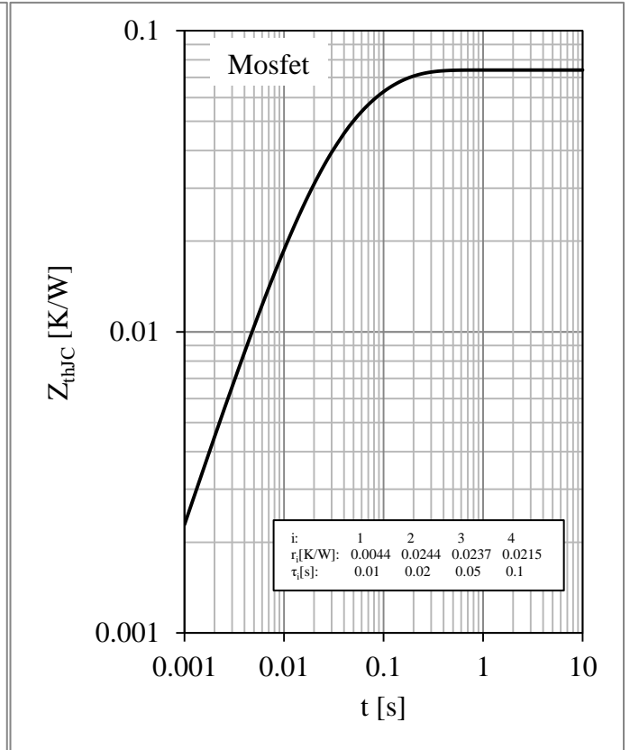
Fig 9. MOSFET Transient Thermal Impedance
